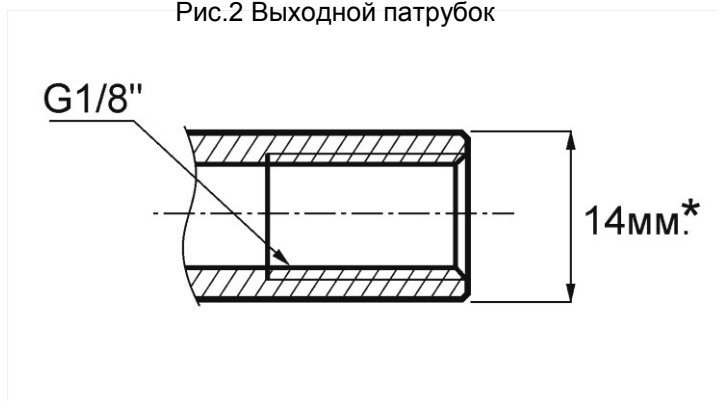
Рис.2 Выходной патрубок
